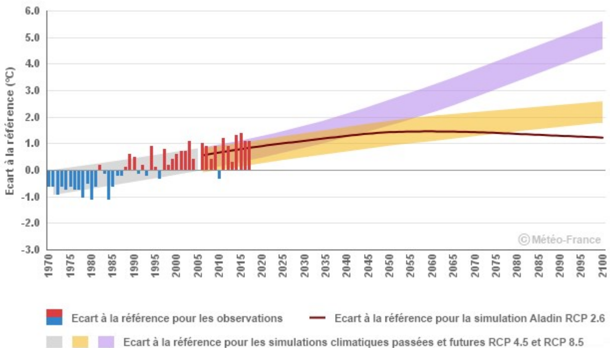
Température moyenne annuelle en Provence-Alpes-Cote d'Azur : écart à la référence 1976-2005 Observations et simulations climatiques pour trois scénarios d'évolution RCP 2.6, 4.5 et 8.5
