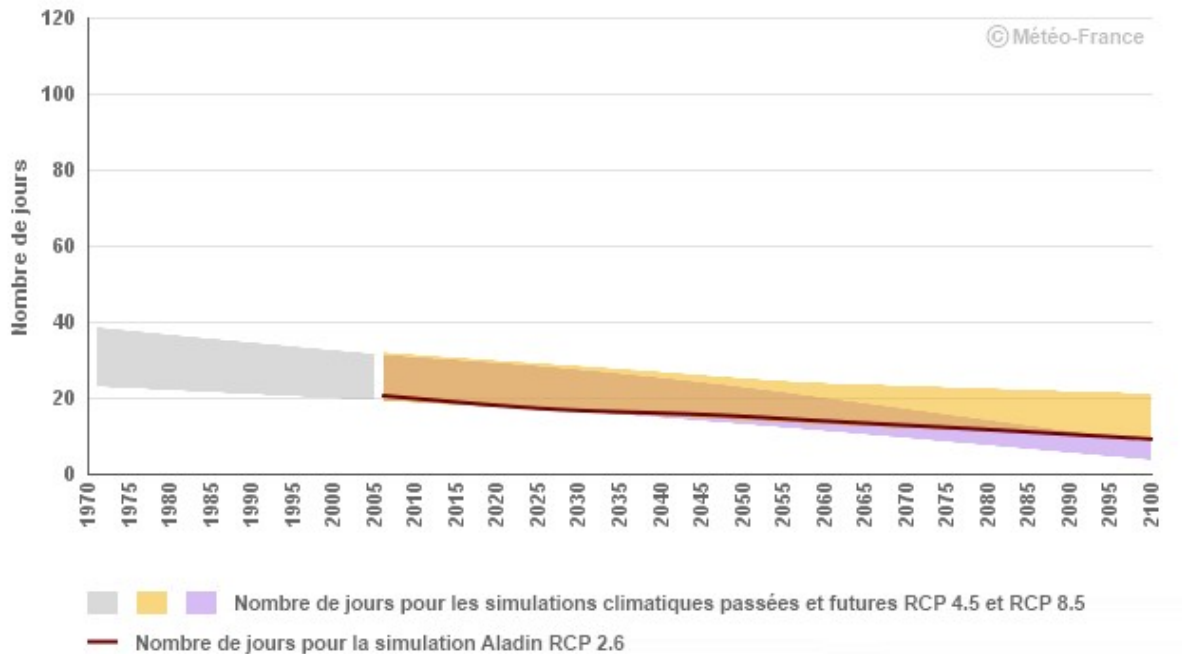
Nombre de jours de gel en Provence-Alpes-Cote d'Azur Simulations climatiques sur passé et futur pour trois scénarios d'évolution RCP 2.6, 4.5 et 8.5
